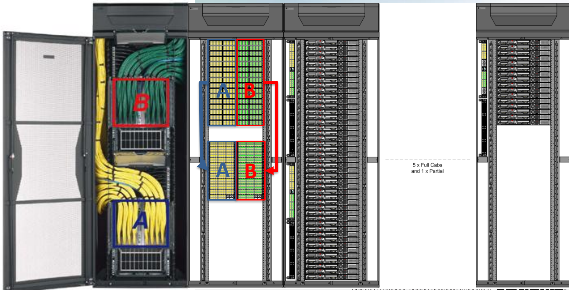
Коммутационный Шкаф
